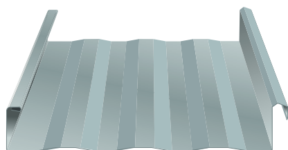
SUPERLOK®
